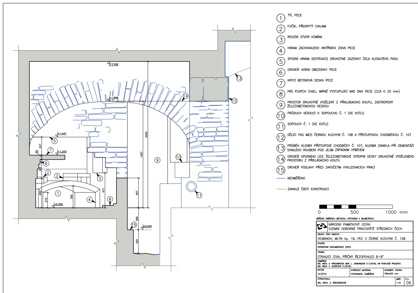
Vicmanov (okres Mladá Boleslav), mlýn čp. 18, operativní dokumentace pece, výkres příčného řezopohledu (zpracovala A. Rákosníková). Na základě provedené dokumentace bude navržen postup obnovy pece, která byla dodatečně vestavěna do prostoru bývalé černé kuchyně.
