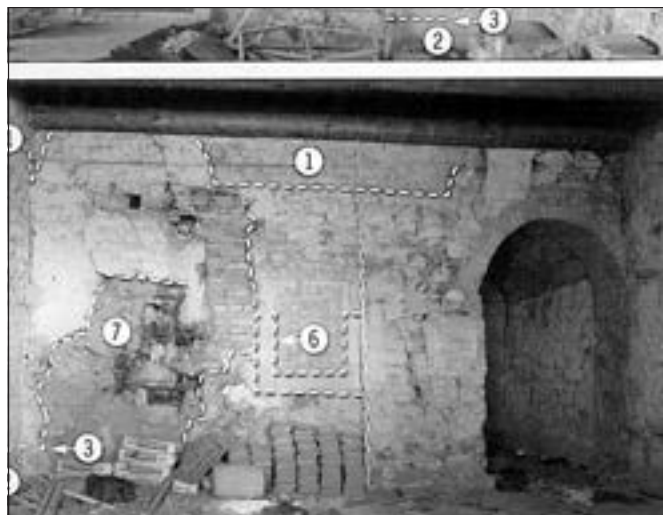
Brandýs nad Labem (okres Praha-východ), dům čp. 98. Pohled na stěnu přední místnosti v přízemí, s otisky odsekanců výběhů klenby s koutovými výsečemi a druhotnými zásabami, souvisejícími s provozem černé kuchyně. Průzkum s dokumentací nálezových situací ve stěnách umožnil nejen rozpoznat jednotlivé etapy stavebního vývoje, ale na základě rozboru dispozice a dokumentace otisků zaniklých klenb a architektonických článků také přiblížit podobu původního pozdně renesančního domu. Pro zhodnocení jeho významu byla právě dokumentace otisků po zaniklých konstrukcích klíčová (foto E. Vyletová).
