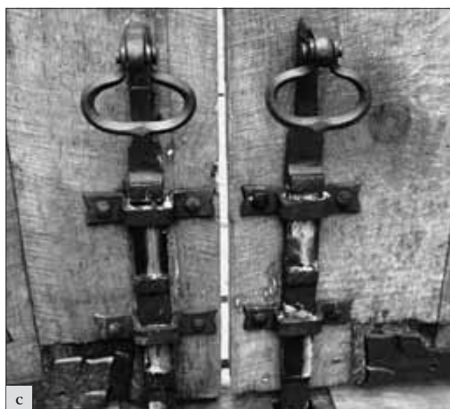
Krakovec (okres Rakovník), brad. Tesařské dohotovení vstupní brány bradu: a – celkový pohled, b, c – detaily kování (foto J. Šobek).
