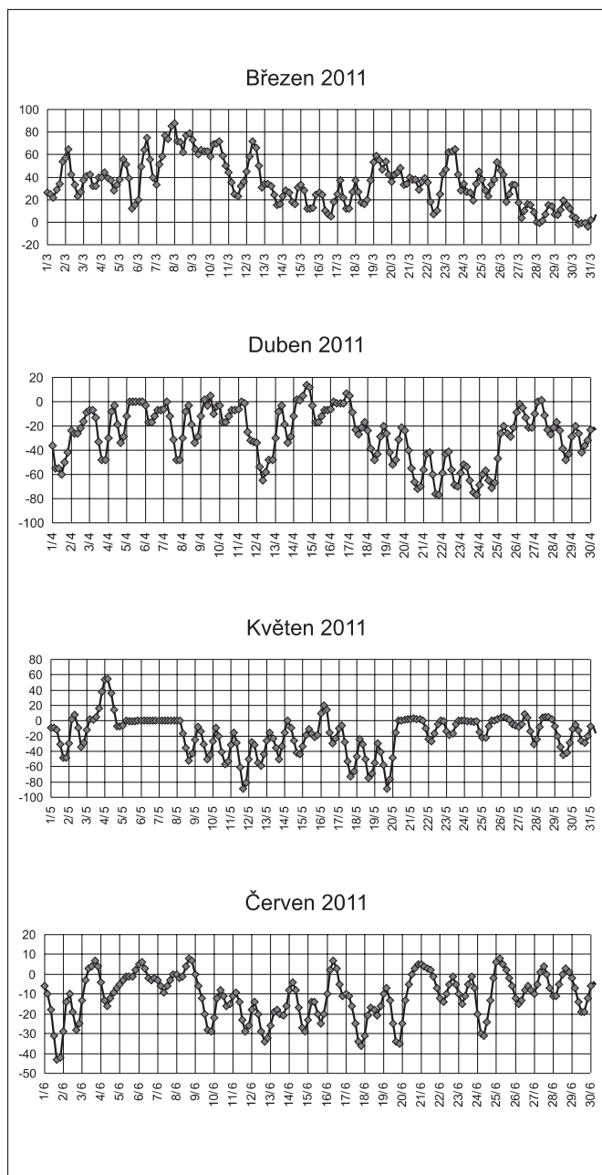
Část výsledku měření proudění v komínu Velké věže na hradě Karlštejn.
