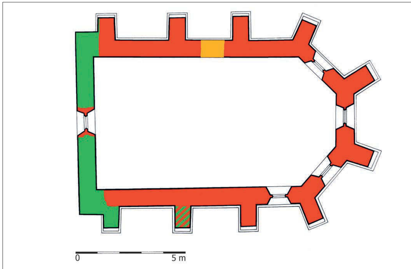
Obr. 6: Markovice, kostel sv. Marka, půdorys v úrovni oken. Červeně: dochované gotické zdivo; zeleně: zdivo z roku 1829; oranžově: zazdívka staršího otvoru z roku 1860; červeno-zeleně: zdivo nejisté doby vzniku (zaměření 2019, 2023; kresba D. Prix, 2023).
