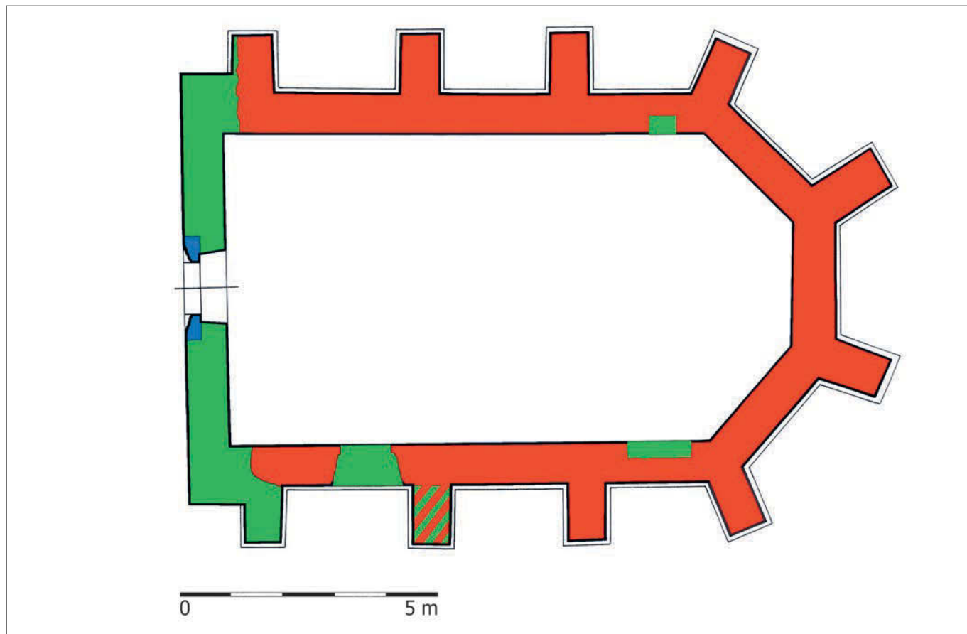
Obr. 5: Markovice, kostel sv. Marka, půdorys v úrovni vstupu. Červeně: dochované gotické zdivo; modře: přenesený renesanční portál; zeleně: zdivo z roku 1829; červeno-zeleně: zdivo nejisté doby vzniku (zaměření 2019, 2023; kresba D. Prix, 2023).
